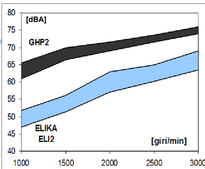
Confronto rumorosità [dBA] pompe Marzocchi: GHP 2 – ELIKA ELI 2 di medesima cilindrata 17.8 cm 3 /giro.
