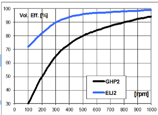
Confronto rendimenti volumetrici a basso numero di giri: pompe Marzocchi: GHP 2 – ELIKA ELI 2 di medesima cilindrata 17.8 cm 3 /giro; P = 200 bar.
